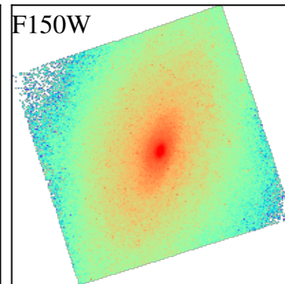
NGC3521
