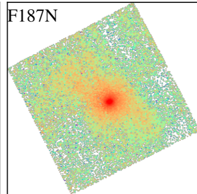
NGC4548
