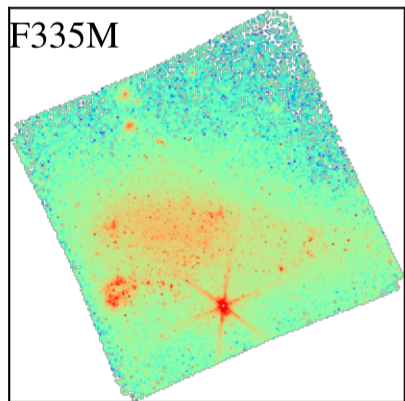
NGC3239
