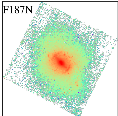
NGC1068
