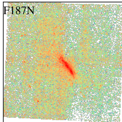
NGC3059
