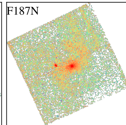
NGC3507
