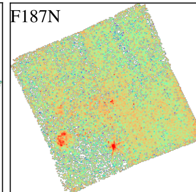
NGC3239
