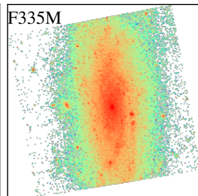
NGC3137
