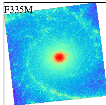
NGC2997
