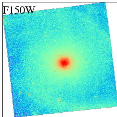
NGC2997
