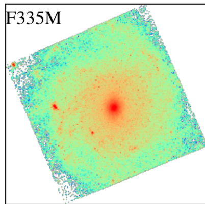
NGC3344
