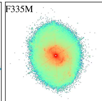
NGC1068
