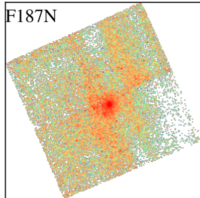
NGC3596
